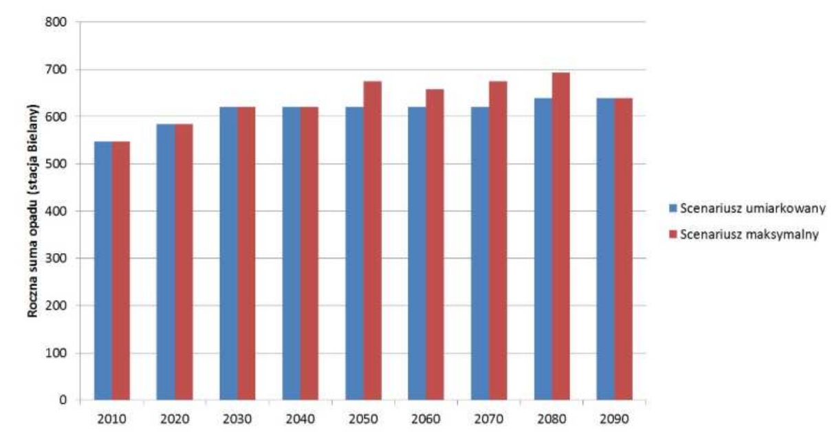
Rysunek 5. Prognozowane sumy roczne opadów atmosferycznych do 2090
